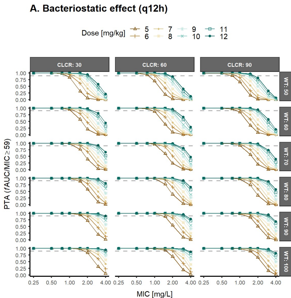
Figura 4.28. (A) Efecto bacteriostático: Probabilidad de alcanzar el efecto bacteriostático objetivo (PTA) ( AUC_{libre}/CMI mayor o igual a 59) tras la administración de una dosis de daptomicina cada 12h a los pacientes con valores de aclaramiento de creatinina y peso corporal indicados; (B) Evaluación de la seguridad: probabilidad de que la concentración mínima de daptomicina sea mayor o igual a 24,3 mg/L.
