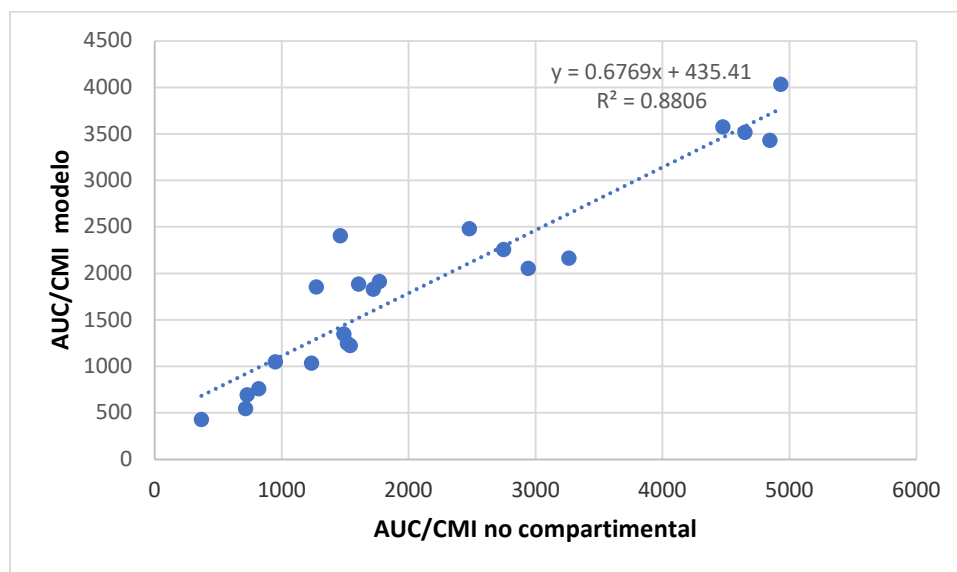
Figura 4.23. Relación entre el AUC/CMI no compartimental y AUC/CMI modelo.
