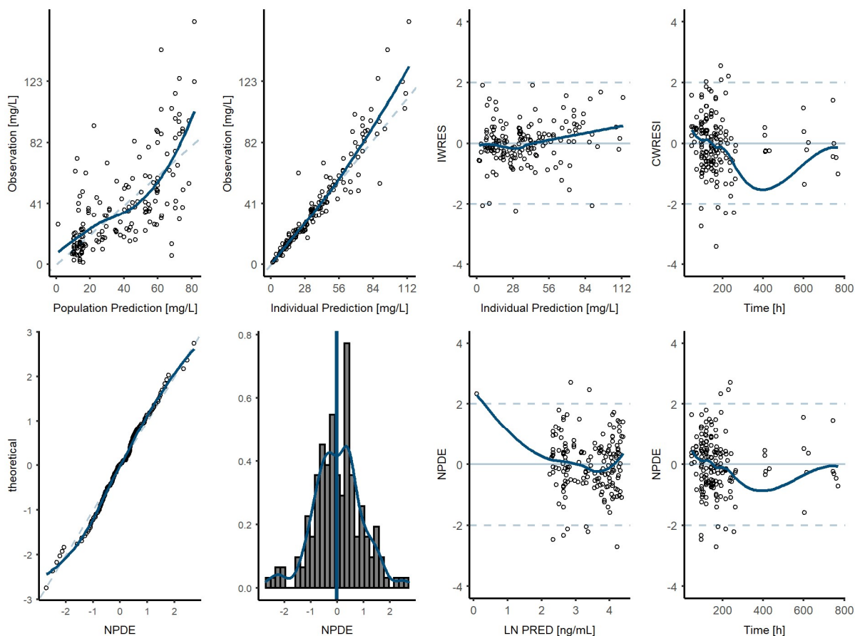
Figura 4.15. Gráficas de bondad de ajuste del modelo farmacocinético estructural base de daptomicina (bicompartimental, PRIOR3).
