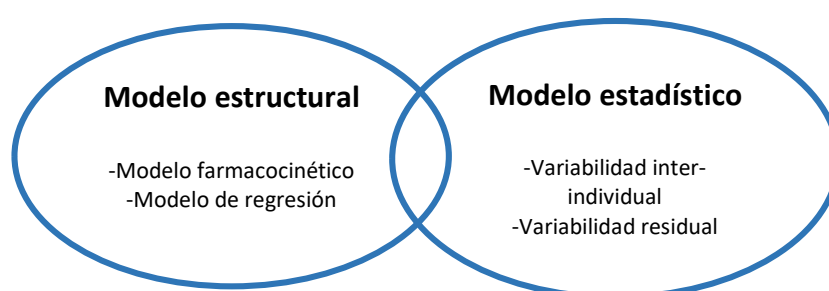
Figura 2.3. Componentes de un modelo farmacocinético.
