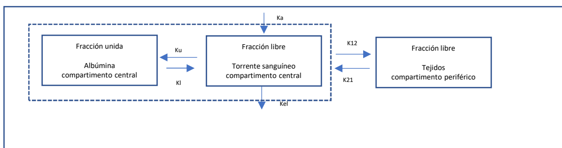
Figura 5.1. Representación del equilibrio del fármaco libre y unido en un modelo bicompartimental. Adaptado de Ulldemolins y col. (65).
