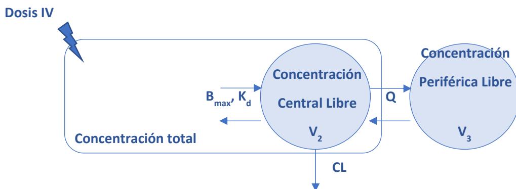
Figura 4.17. Esquema del modelo PK bicompartimental con unión de la daptomicina a las proteínas plasmáticas.
