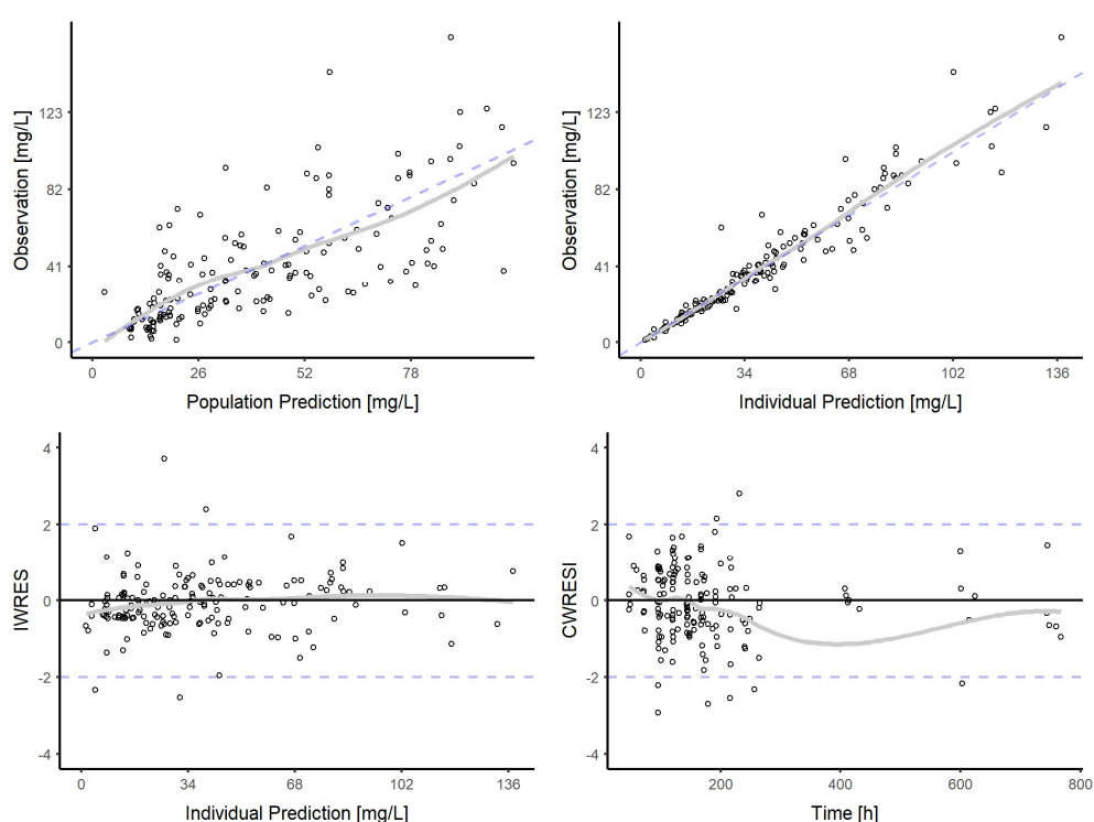
Figura 4.20. Gráficos de bondad de ajuste del modelo farmacocinético poblacional final de daptomicina.
