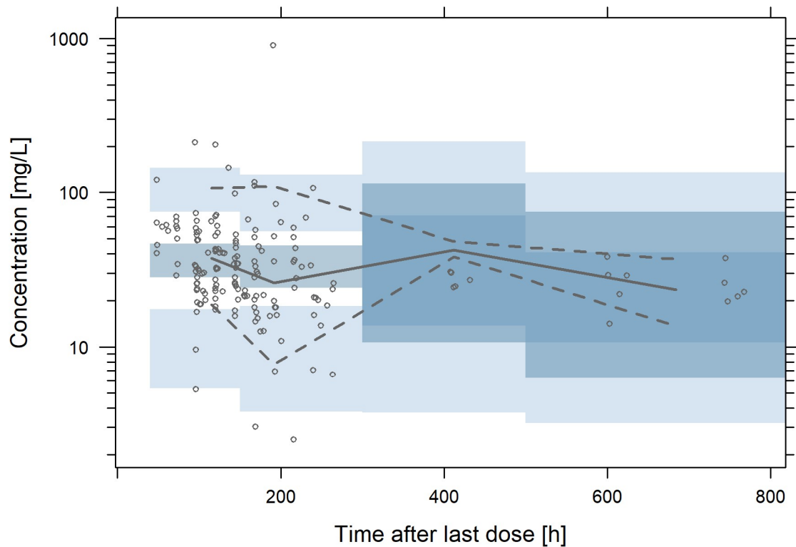
Figura 4.16. VPC del modelo farmacocinético estructural base de daptomicina (bicompartimental, PRIOR3) representado en escala logarítmica.
