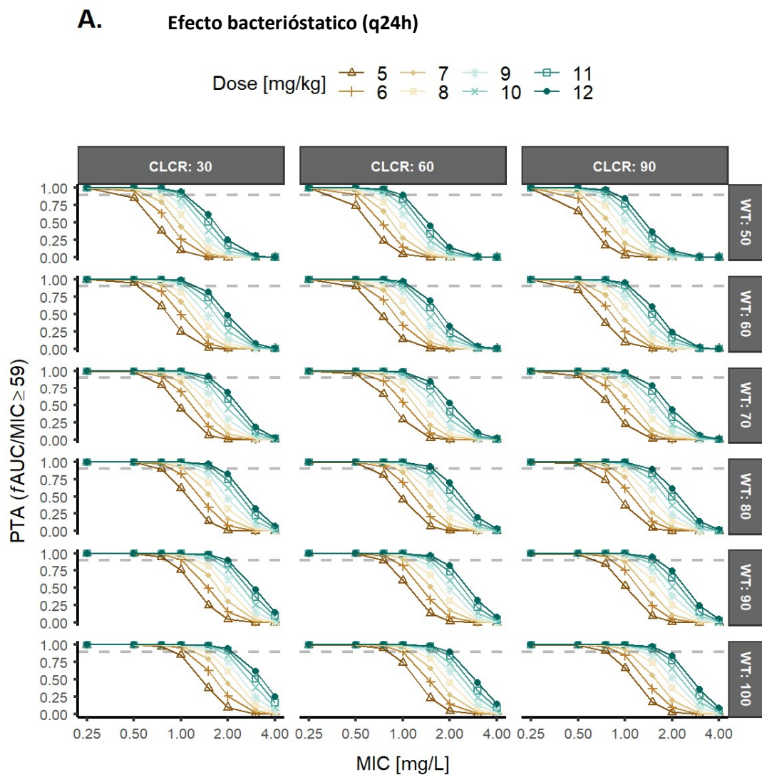
Figura 4.26. (A) Efecto bacteriostático: Probabilidad de alcanzar el objetivo (PTA) (efecto bacteriostático, AUC_{libre}/CMI mayor o igual a 59) tras la administración de una dosis diaria (q24h) de daptomicina en pacientes con valores de aclaramiento de creatinina y peso corporal indicados; (B) Evaluación de la seguridad: probabilidad de que la concentración mínima de daptomicina sea mayor o igual a 24,3 mg/L.
