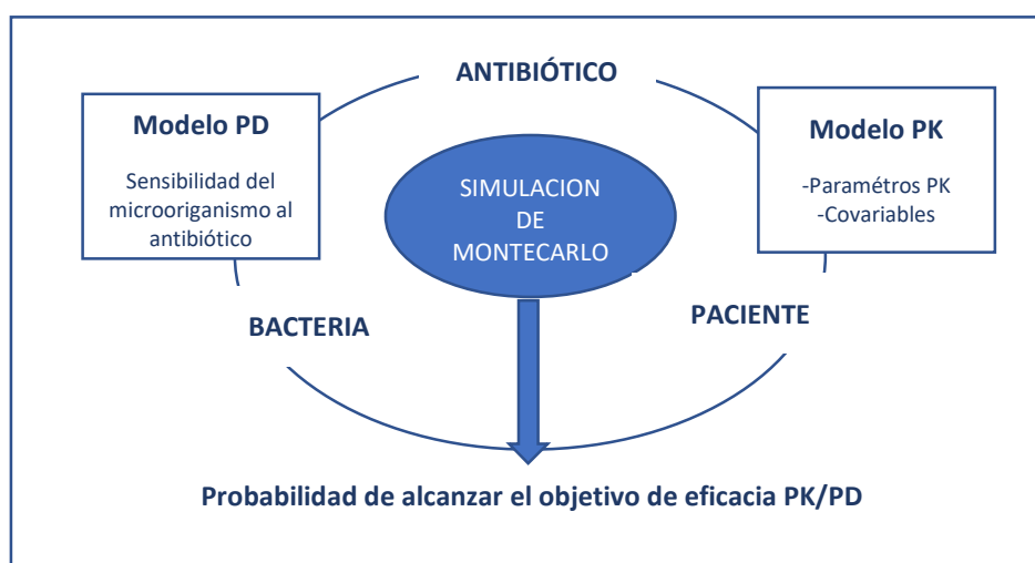
Figura 2.5. Esquema de Simulación de Monte Carlo (adaptado de Canut y col. (29))
