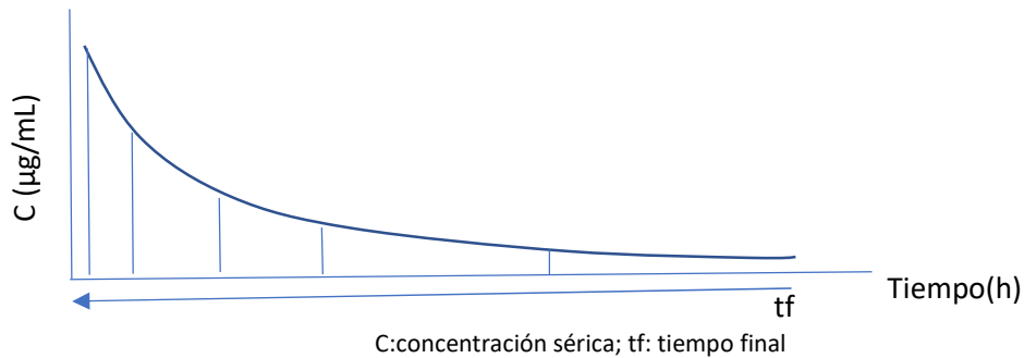
Figura 3.1. Cálculo de AUC por el método de los trapecios.
