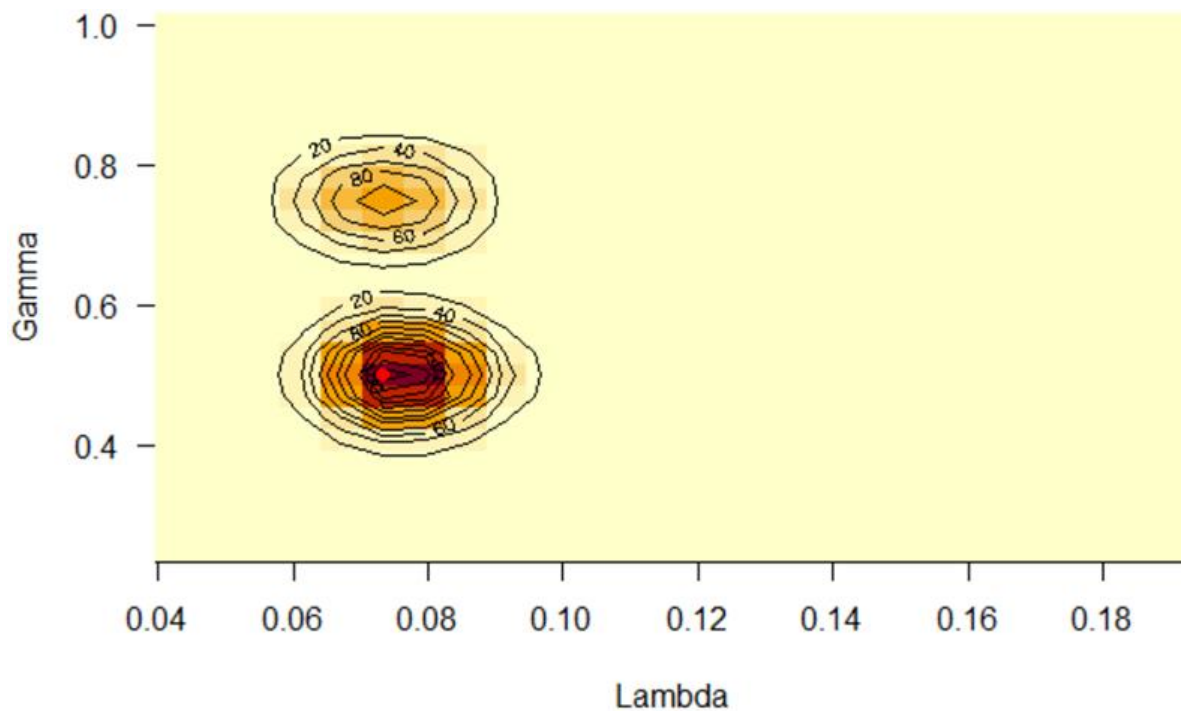
Figura 56: Representación de la gráfica de densidad bidimensional para los posibles valores de los parámetros asociados con la aparición de complicaciones durante o tras la ejecución de los procedimientos, según el modelo de regresión logística penalizada mediante elastic net relajado.
