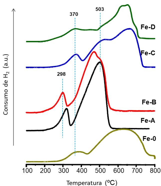
Figura 4.4. Reducción a temperatura programada de los catalizadores de óxido de hierro másicos.
