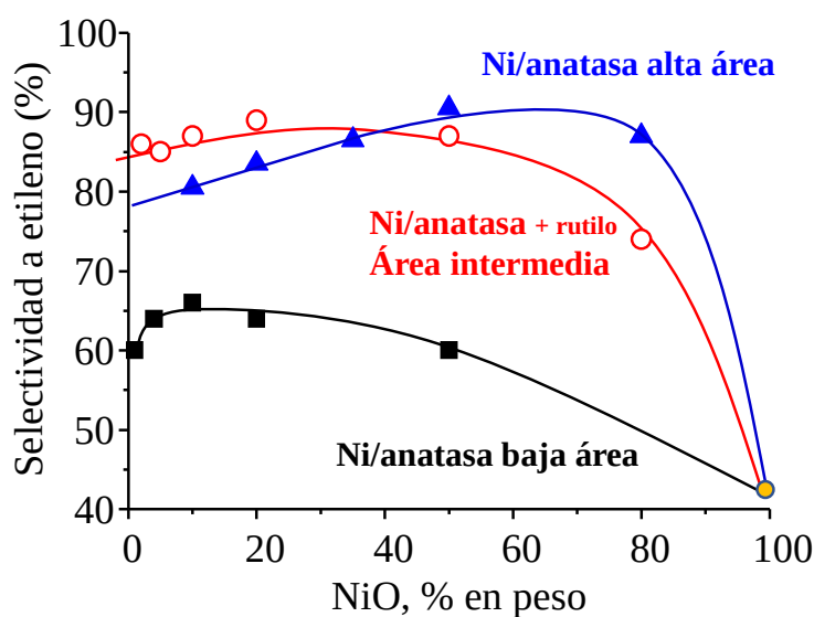
Figura 6. 12. Selectividad a etileno frente al contenido de níquel en los catalizadores soportados en \text{TiO}_2 .
