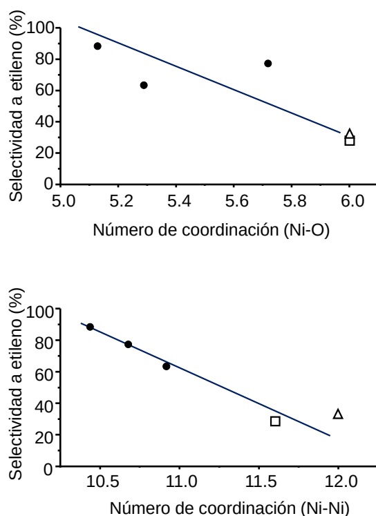
Figura 5.14. Variación de la selectividad a etileno con el número de coordinación Ni-O o Ni-Ni determinados por espectroscopía EXAFS. Nota: Selectividad a etileno a 450°C y una conversión de etano del 10%. Símbolos: Catalizadores con Ti (●), NiO sin soportar (△), NiO/SiO 2 (□).
