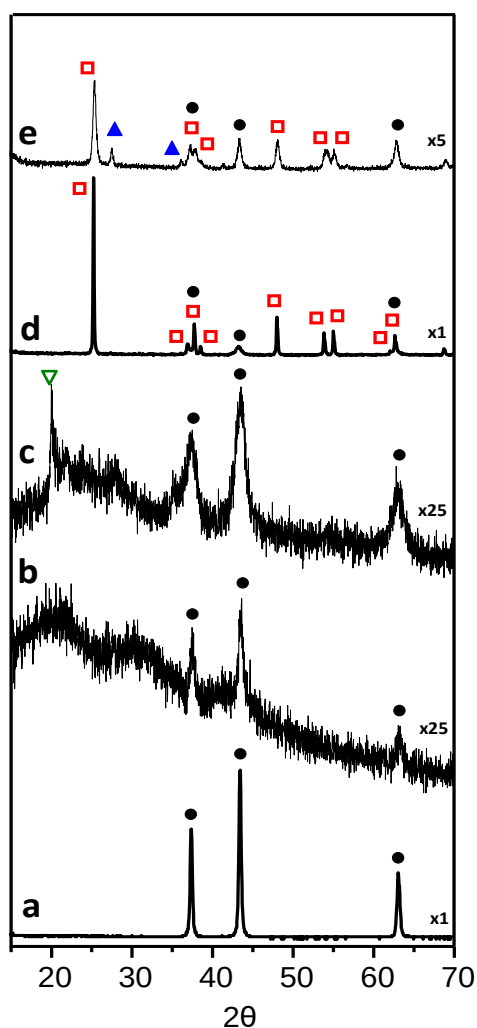
Figura 5.5. Patrones de rayos X de los catalizadores de NiO soportados. a) NiO, b) NiO/SiO 2 , c) NiO/PCH-Ti, d) NiO/Ti-anat, e) NiO/Ti-P25. Símbolos: NiO (●), PCH-Ti (▽), TiO 2 -anatasa (◻), TiO 2 -rutilo (▲).
