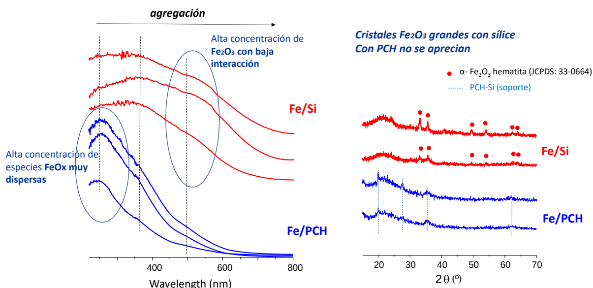
Figura 6.6. Dispersión del óxido de hierro sobre el PCH y sílice convencional (DR-UV-Vis. y DRX).
