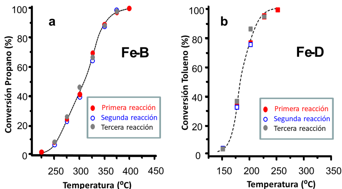
Figura 4.10. Pruebas de estabilidad: a) Variación de la conversión de propano con la temperatura de reacción para el catalizador Fe-B; y b) Variación de la conversión de tolueno con la temperatura de reacción para el catalizador Fe-D. Símbolos: (●, ■) 1 er ciclo, (○, □) 2 o ciclo, (●, ■) 3 er ciclo. Nota: Condiciones de reacción en el texto.
