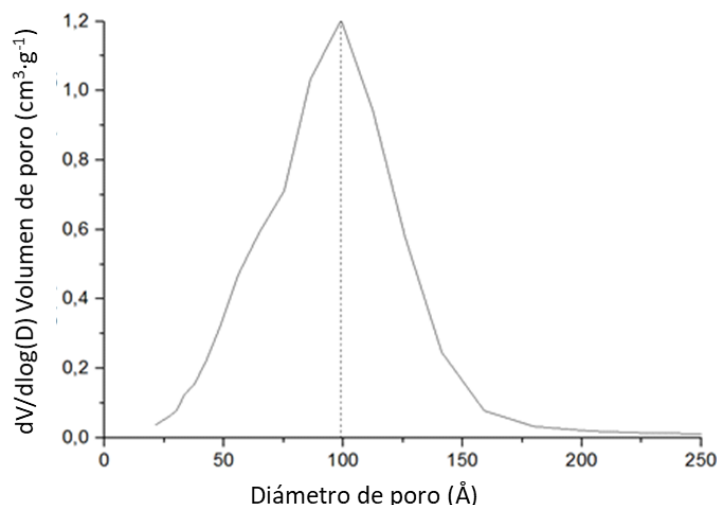
Figura 4.2. Distribución de poro del catalizador Fe-D.
