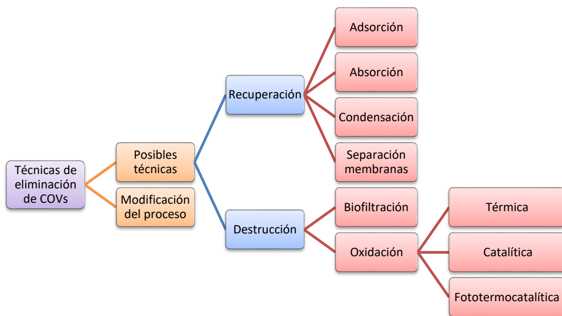
Figura 1.1. Técnicas de eliminación de COVs.
