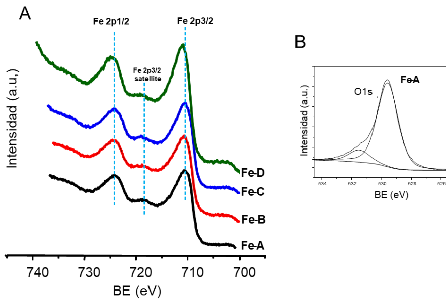
Figura 4.5. Espectros XPS Fe 2p para los catalizadores de óxido de hierro sintetizados (A) y deconvolución de la señal O1s (B).
