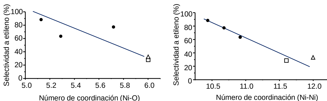
Figura 6. 11. Variación de la selectividad a etileno con el número de coordinación Ni-O o Ni-Ni determinados por espectroscopía EXAFS. Nota: Selectividad a etileno a 450°C y una conversión de etano del 10%. Símbolos: Catalizadores con Ti (●), NiO sin soportar (△), NiO/SiO 2 (□).
