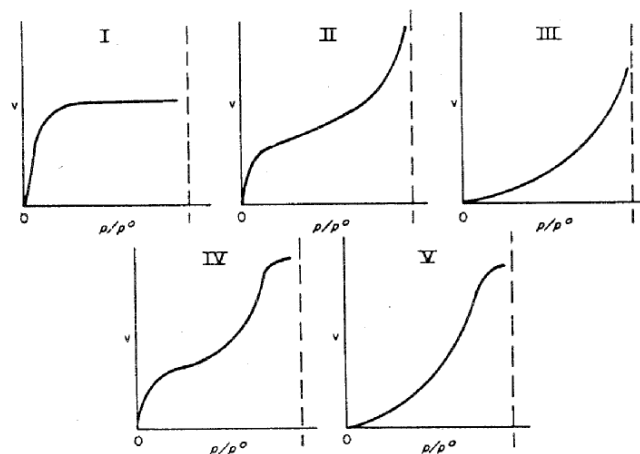
Figura 3.4. Tipos de isothermas de adsorción según la clasificación de Brunauer
