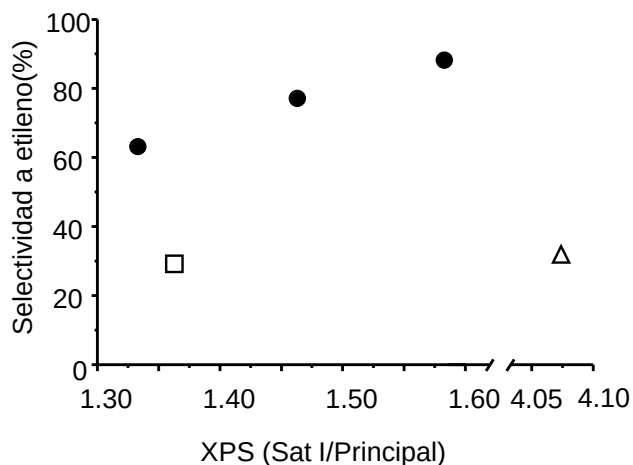
Figura 5.12. Relación entre la selectividad a etileno y el cociente Satélite I/Principal (Ni 2p 3/2 core level por XPS). Símbolos: Catalizadores con titanio (●), NiO sin soportar (Δ), NiO/SiO 2 (◻).
