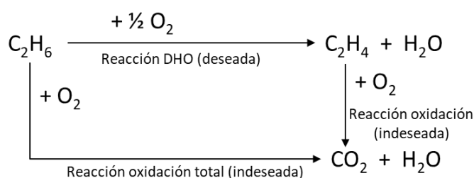
Figura 1.8. Posibles reacciones que tienen lugar en la DHO de etano usando catalizadores. Nota: con la mayoría de los catalizadores se forma CO además de CO 2 .
