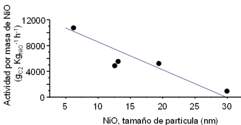
Figura 5.6. Influencia del tamaño de cristal del NiO sobre la actividad catalítica. Nota; Condiciones de reacción en Tabla 5.1.
