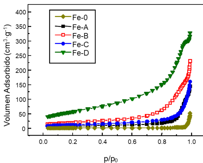
Figura 4.1. Isotermas de adsorción para los catalizadores de óxido de hierro preparados por diferentes métodos.
