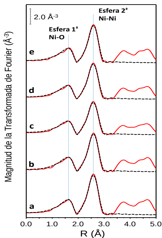
Figura 5.13. Transformada de Fourier de los espectros EXAFS (región Ni K-edge) de los catalizadores de NiO soportados y sin soportar. Catalizadores: a) NiO, b) NiO/SiO 2 , c) NiO/PCH-Ti, d) NiO/Ti-anat, and e) NiO/Ti-P25.
