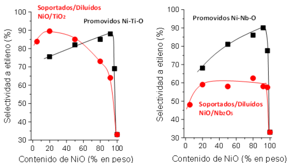
Figura 6. 15. Comparativa de selectividad a etileno frente al contenido de NiO entre catalizadores soportados/diluídos frente a promovidos para los diferentes soportes de Ti y Nb. 450°C y 10% de conversión.
