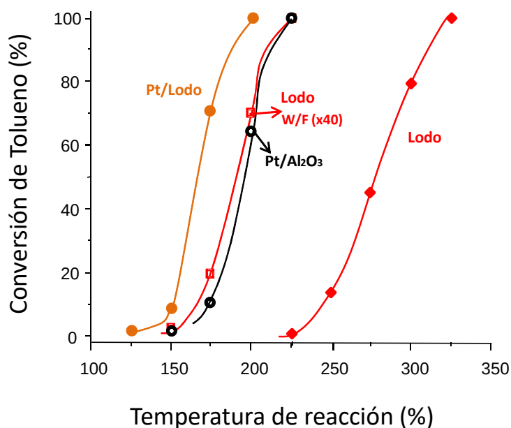
Figura 6.7. Conversión de tolueno frente a la temperatura de reacción en la oxidación total, para los catalizadores empleados (Lodo, Pt/Lodo y Pt/alumina). Condiciones de reacción en el capítulo correspondiente.
