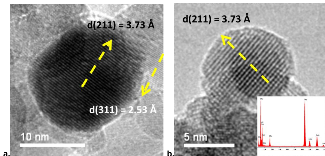
Figura 4.7. Imágenes de alta resolución de partículas de \alpha\text{-Fe}_2\text{O}_3 , (a) Fe-C, (b) Fe-D. La figura insertada en (b) es el espectro correspondiente del EDX del área seleccionada.
