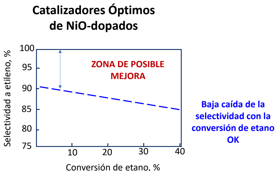
Figura 5.3. Selectividad a etileno frente a la conversión de etano para un catalizador óptimo de NiO dopado.
