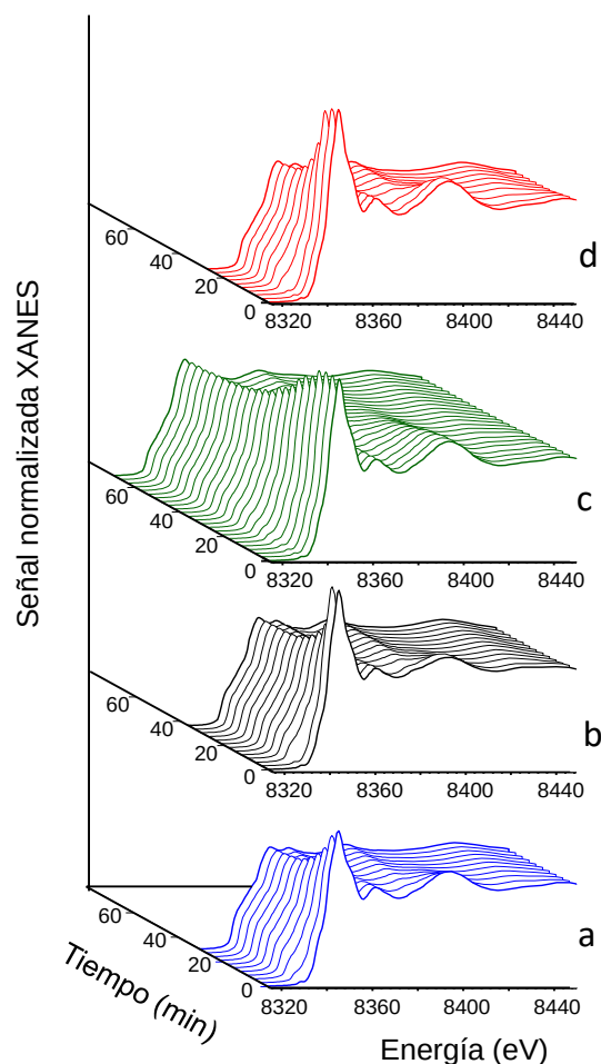
Figura 5.9. Evolución con el tiempo de los espectros XANES (en la región de Ni K-edge) durante la reducción en atmósfera de \text{H}_2 de catalizadores de níquel: a) NiO, b) NiO/SiO 2 , c) NiO/PCH-Ti, y d) NiO/Ti-P25. Condiciones de reducción: T=450\text{ }^\circ\text{C} ; \text{H}_2/\text{He} , 25/25 ( \text{mL min}^{-1} ).
