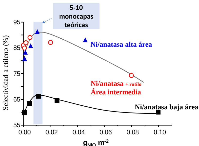
Figura 6.14. Selectividad a etileno para los distintos soportes en función de la masa de \text{NiO} por \text{m}^2 de área de soporte
