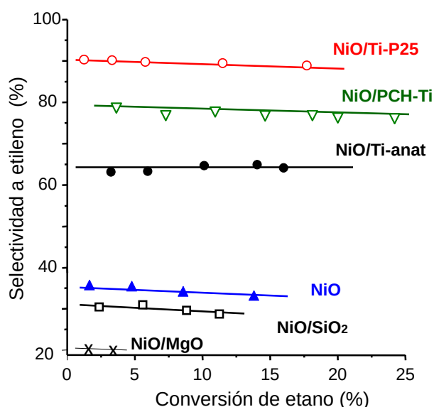
Figura 5.4. Variación de la selectividad a etileno con la conversión de etano usando catalizadores de NiO soportados. Símbolos: NiO ( \blacktriangle ), NiO/MgO ( \times ), NiO/SiO 2 ( \blacksquare ), NiO/PCH-Ti ( \nabla ), NiO/Ti-anat ( \bullet ), NiO/Ti-P25 ( \circ ). Condiciones de reacción detalladas en el texto.
