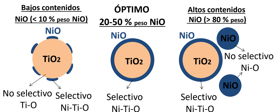
Figura 6.13. Influencia del contenido de níquel en catalizadores de NiO soportados en \text{TiO}_2 sobre la selectividad a etileno.
