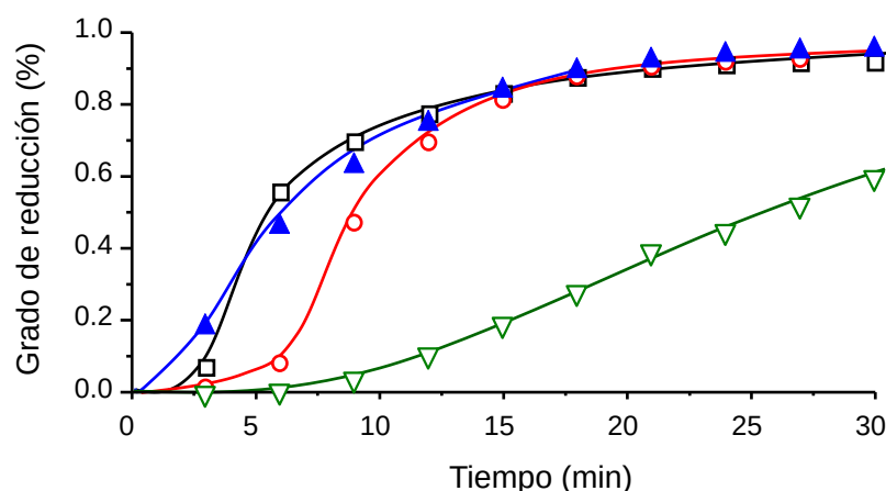
Figura 6.10. Curvas cinéticas de reducción en H 2 calculadas por ajustes lineales de los espectros XANES (en la región de Ni K-edge). Condiciones de reducción: T=450 °C; H 2 /He, 25/25 (mL min -1 ). Símbolos: NiO (▲), NiO/SiO 2 (■), NiO/PCH-Ti (▼), NiO/Ti-P25 (●). Un grado de reducción 0 implica un estado de oxidación de níquel de 2 (Ni 2+ ) y un grado de reducción 1 implica un estado de oxidación 0 (Ni 0 ).
