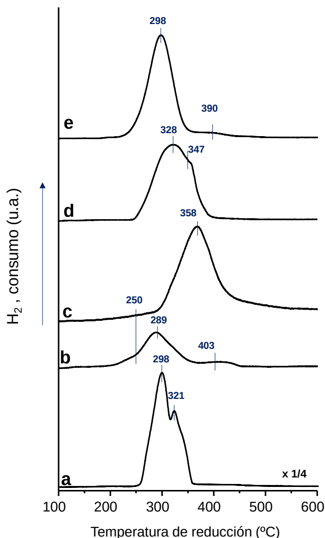
Figura 5.7. Reducción a temperatura programada ( H_2 -TPR) de los catalizadores de NiO soportados y sin soportar. a) NiO, b) NiO/SiO 2 , c) NiO/PCH-Ti, d) NiO/Ti-anat, y e) NiO/Ti-P25.
