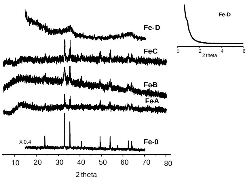
Figura 4.3. Patrones de DRX para catalizadores de óxidos de hierro. También se ha incluido el patrón DRX de bajo ángulo para Fe-D.
