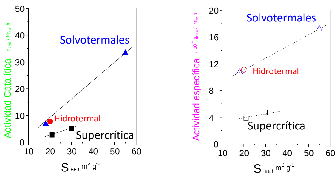
Figura 6.4. Actividad catalítica y actividad normalizada por el área del catalizador frente al área superficial, para los catalizadores preparados en agua supercrítica, por métodos hidrotermales y solvotermales.
