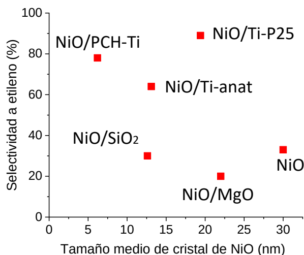
Figura 6. 9. Relación entre el tamaño de cristal de NiO y la selectividad a etileno. Notas: Selectividad a etileno para una conversión del 10% y 450°C. Tamaño medio de cristal estimado por DRX mediante la ecuación de Scherrer. Otras condiciones de reacción en el texto.
