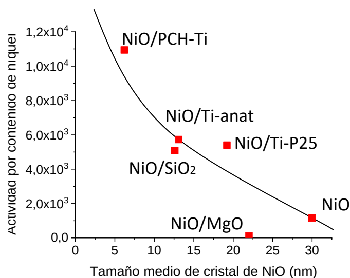
Figura 6.8. Relación entre el tamaño de cristal de NiO y la actividad catalítica normalizada por el contenido de NiO. Notas: Actividad catalítica a 450 °C y conversiones inferiores al 5% en \text{gC}_2\text{H}_6 \text{ kgNiO}^{-1} \text{ h}^{-1} . Tamaño medio de cristal estimado por DRX mediante la ecuación de Scherrer.
