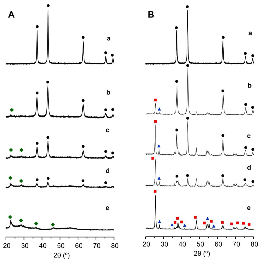
Figure S3. XRD patterns of Nb 2 O 5 - (A) and TiO 2 -P25- (B) diluted NiO catalysts. a) NiO; b) 80NiO/Nb 2 O 5 , 80NiO/TiO 2 ; c) 50NiO/Nb 2 O 5 , 50NiO/TiO 2 ; d) 50NiO/Nb 2 O 5 , 20NiO/TiO 2 ; e) Nb 2 O 5 , TiO 2 . Symbols: (●) NiO; (◆) Nb 2 O 5 ; (▲) TiO 2 -rutile; (■) TiO 2 -anatase
