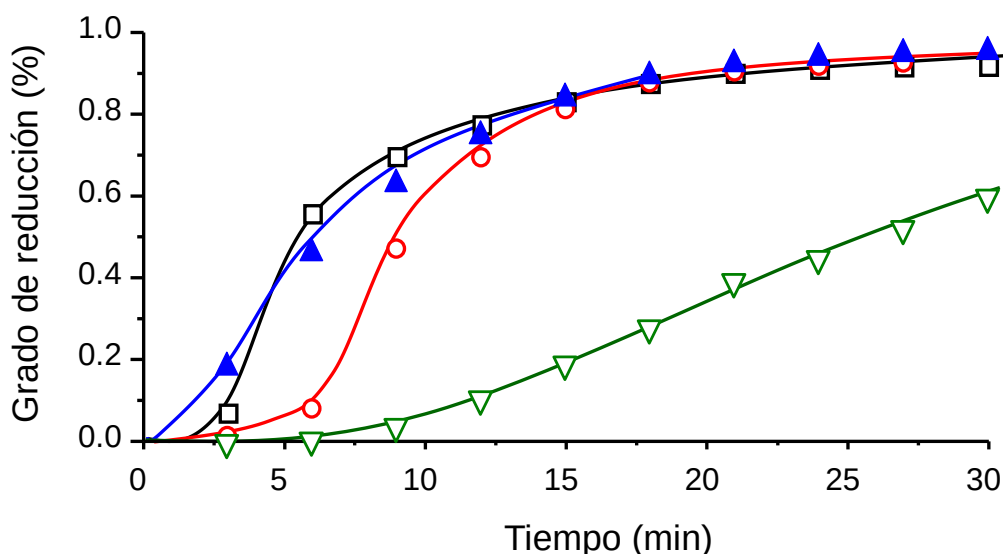
Figura 5.10. Curvas cinéticas de reducción en H_2 calculadas por ajustes lineales de los espectros XANES (en la región de Ni K-edge). Condiciones de reducción: T=450\text{ }^{\circ}\text{C} ; H_2/He , 25/25 ( \text{mL min}^{-1} ).. Symbols: NiO (▲), NiO/SiO 2 (■), NiO/PCH-Ti (▼), NiO/Ti-P25 (●) .
