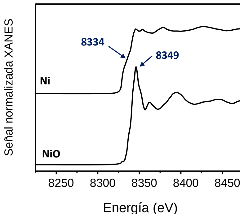
Figura 5.8. Espectros XANES normalizados de NiO y Ni puros.
