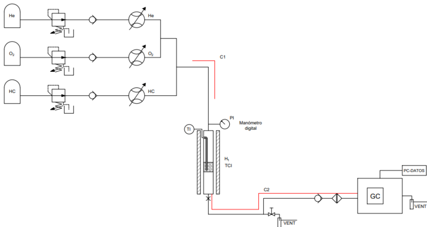
Figura 3. 5. Esquema del sistema de reacción empleado.
