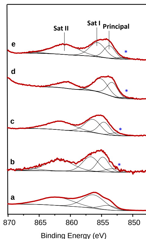
Figura 5.11. Espectro de XPS (Ni 2p 3/2 core level) de los catalizadores de NiO soportados y sin soportar. a) NiO, b) NiO/SiO 2 , c) NiO/PCH-Ti, d) NiO/Ti-anat, y e) NiO/Ti-P25.
