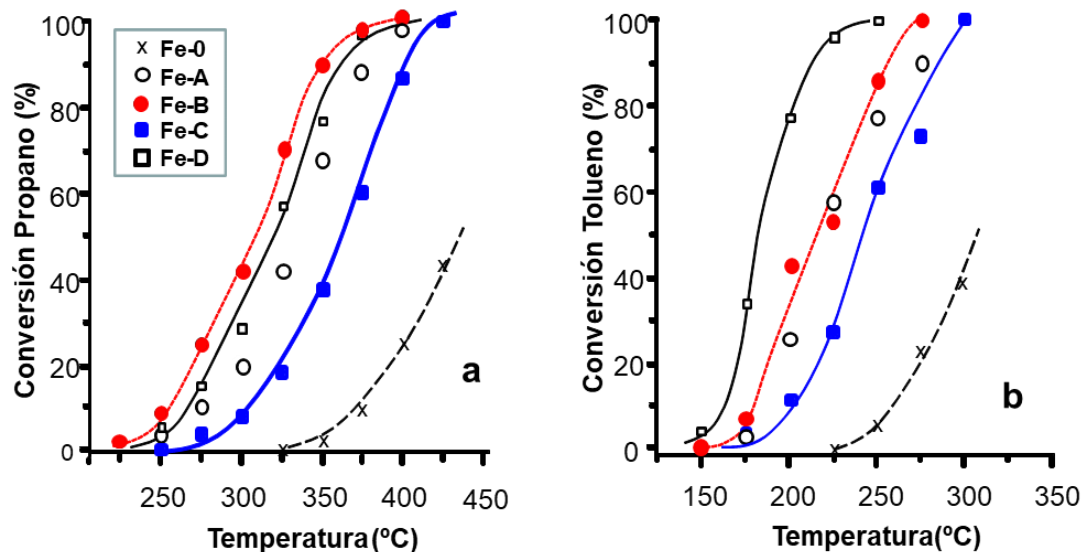
Figura 4.8. Variación de la conversión de propano (a) y tolueno (b) con la temperatura de reacción para los catalizadores de óxido de hierro preparados de manera diferente. Símbolos: (x) Fe-0, (O) Fe-A, (●) Fe-B, Fe-C (■), Fe-D (□). Nota: GHSV=30000h -1 , las condiciones de reacción se muestran en el texto.
