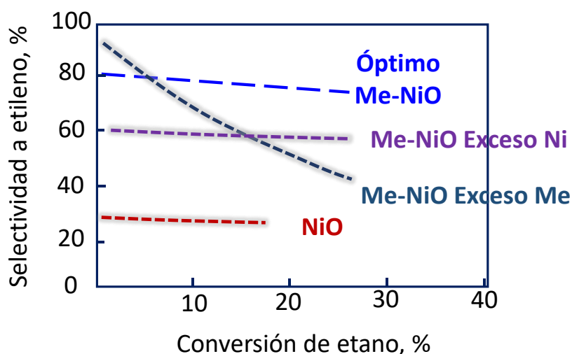
Figura 5.1. Selectividad a etileno frente a conversión de etano para un catalizador basado en óxido de níquel y este con diferentes cantidades de promotor.
