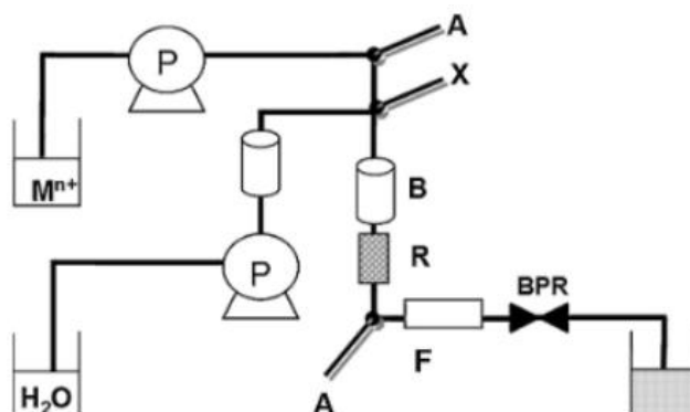
Figura 3. 1. Esquema del montaje experimental hidrotermal. A: sensores de presión, X: punto de mezcla, B: calentador y reactor, P: bombas, F: filtro (2 m), BPR: regulador de contrapresión ("Tescom")
