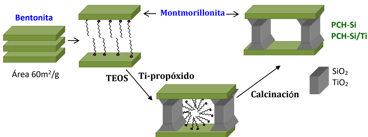
Figura 3.2. Síntesis de arcilla pilareada de Silicio (PCH-Si) y arcilla pilareada de Silicio y Titanio (PCH-Si/Ti).
