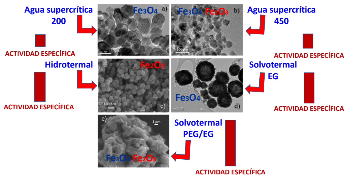
Figura 6.5. Microcopía electrónica de barrido (SEM), mostrando las diferentes fases \text{Fe}_3\text{O}_4 y \text{Fe}_2\text{O}_3 y la actividad específica para los catalizadores de óxido de hierro preparados por el proceso; a) agua supercrítica a 200°C, b) agua supercrítica a 450°C, c) hidrotermal, d) solvotermal con etilenglicol y e) solvotermal con polietilenglicol/etilenglicol.
