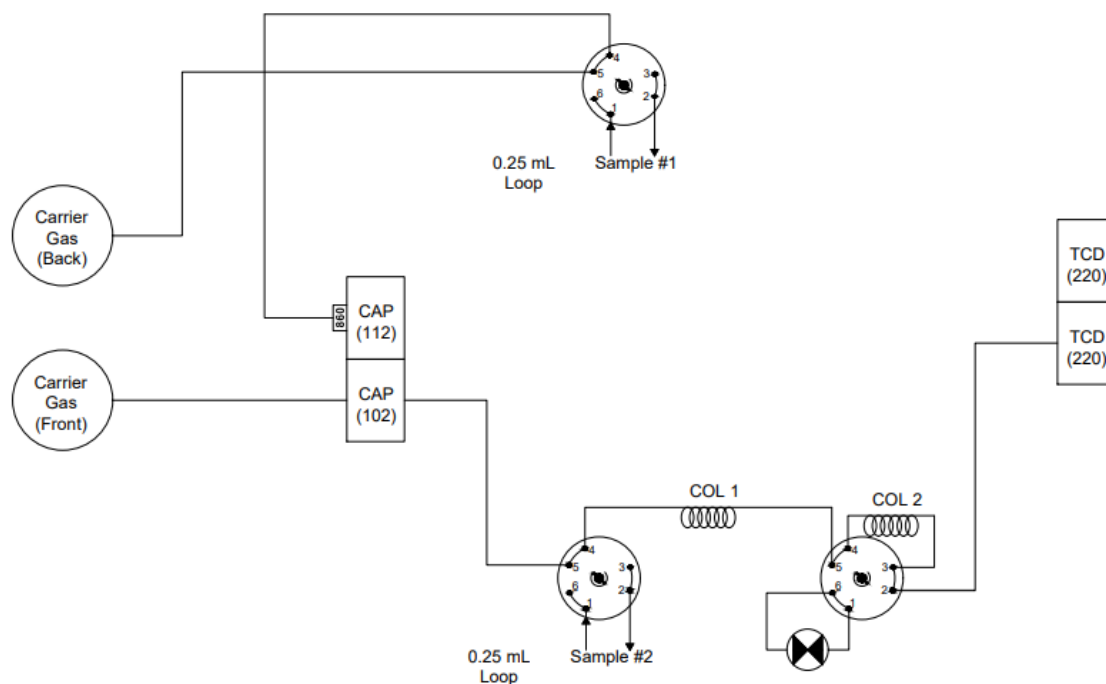
Figura 3.7. Esquema del sistema de inyección (funcionamiento del cromatógrafo de gases).
