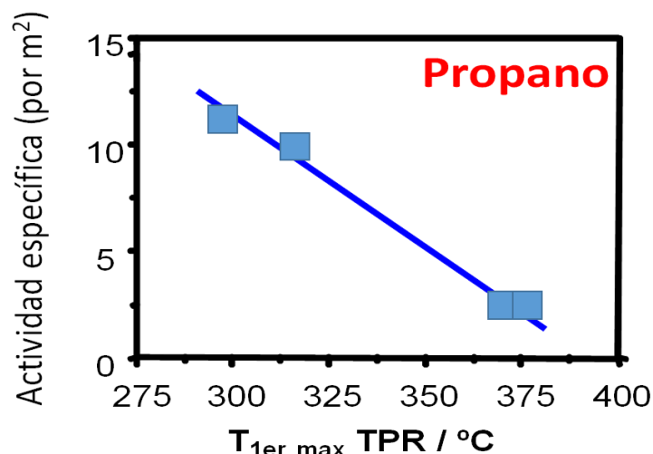
Figura 6.2. Influencia de la temperatura de reducción (máximo del primer pico observado por TPR) sobre la actividad específica de los diferentes óxidos de hierro en la oxidación total de propano.
